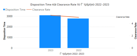
Γράφημα 11: Μικροδιαφορές
