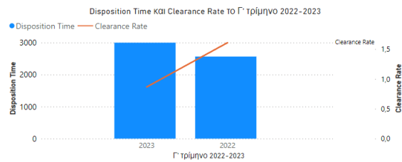
Γράφημα 7: Εργατικά/Αμοιβές
